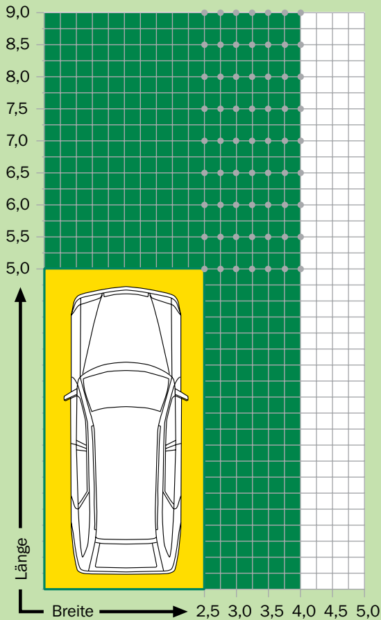
Die Draufsicht zeigt, in welchen Breiten und Längen der Carport ausgeführt werden kann.
